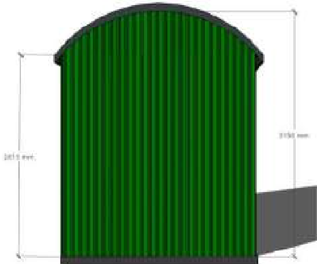
RHS ELEVATION
