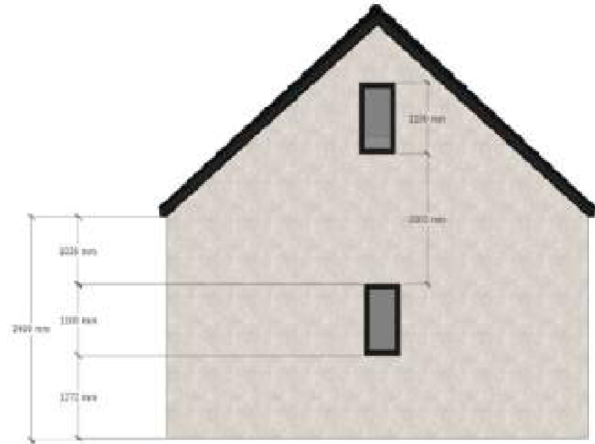
RHS ELEVATION
