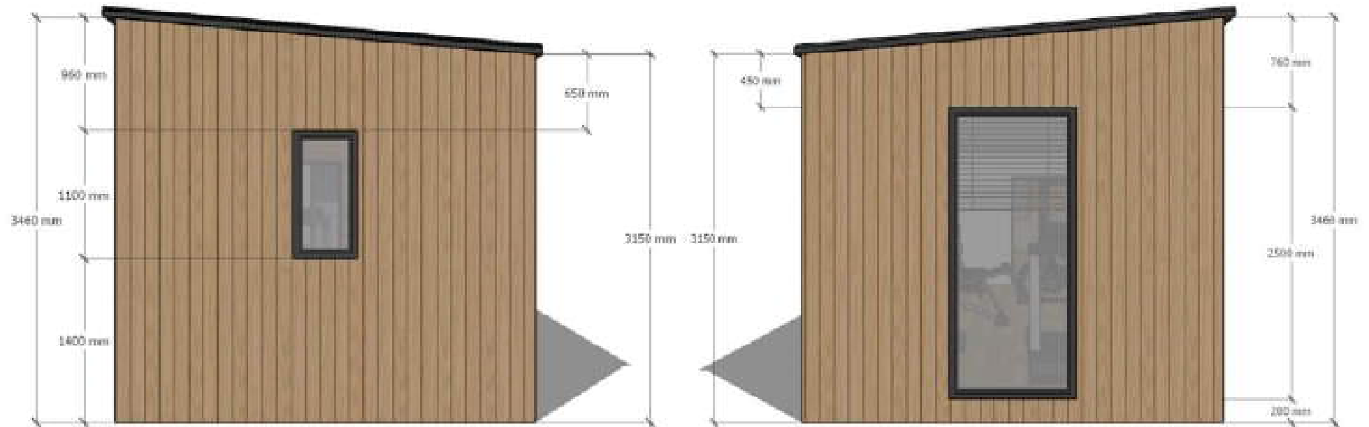
RHS ELEVATION
