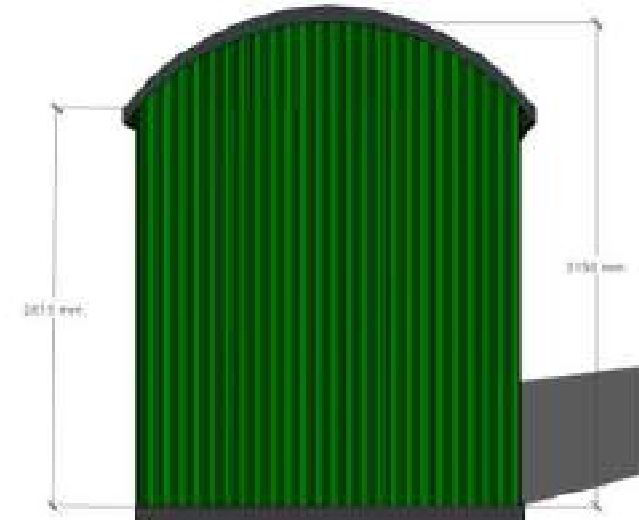
RHS ELEVATION
