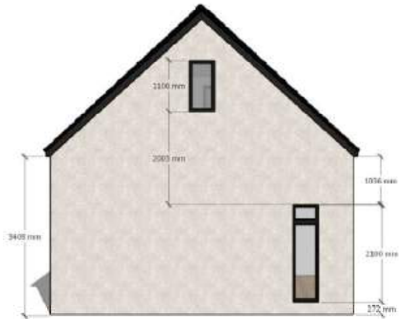
RHS ELEVATION
